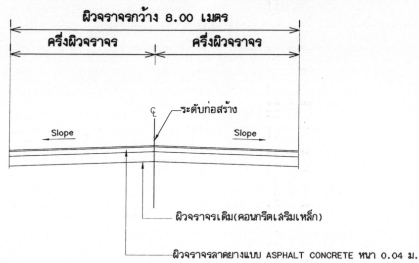
รูปตัดแสดงโครงสร้างถนนและคุณสมบัติวัสดุ ไม่แสดงมาตราส่วน
